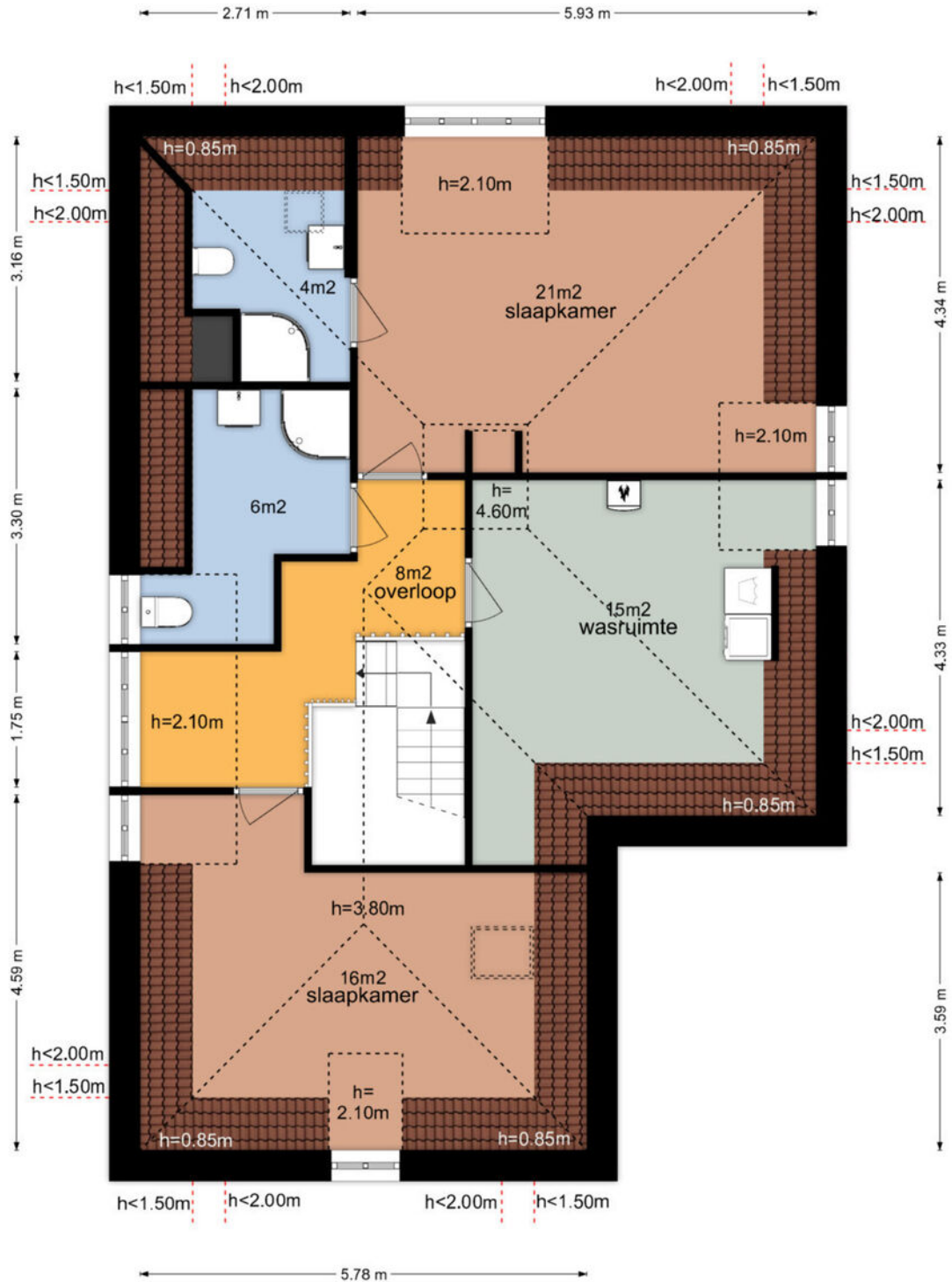
Ten Katelaan 10 - Bilthoven Tweede Verdieping
