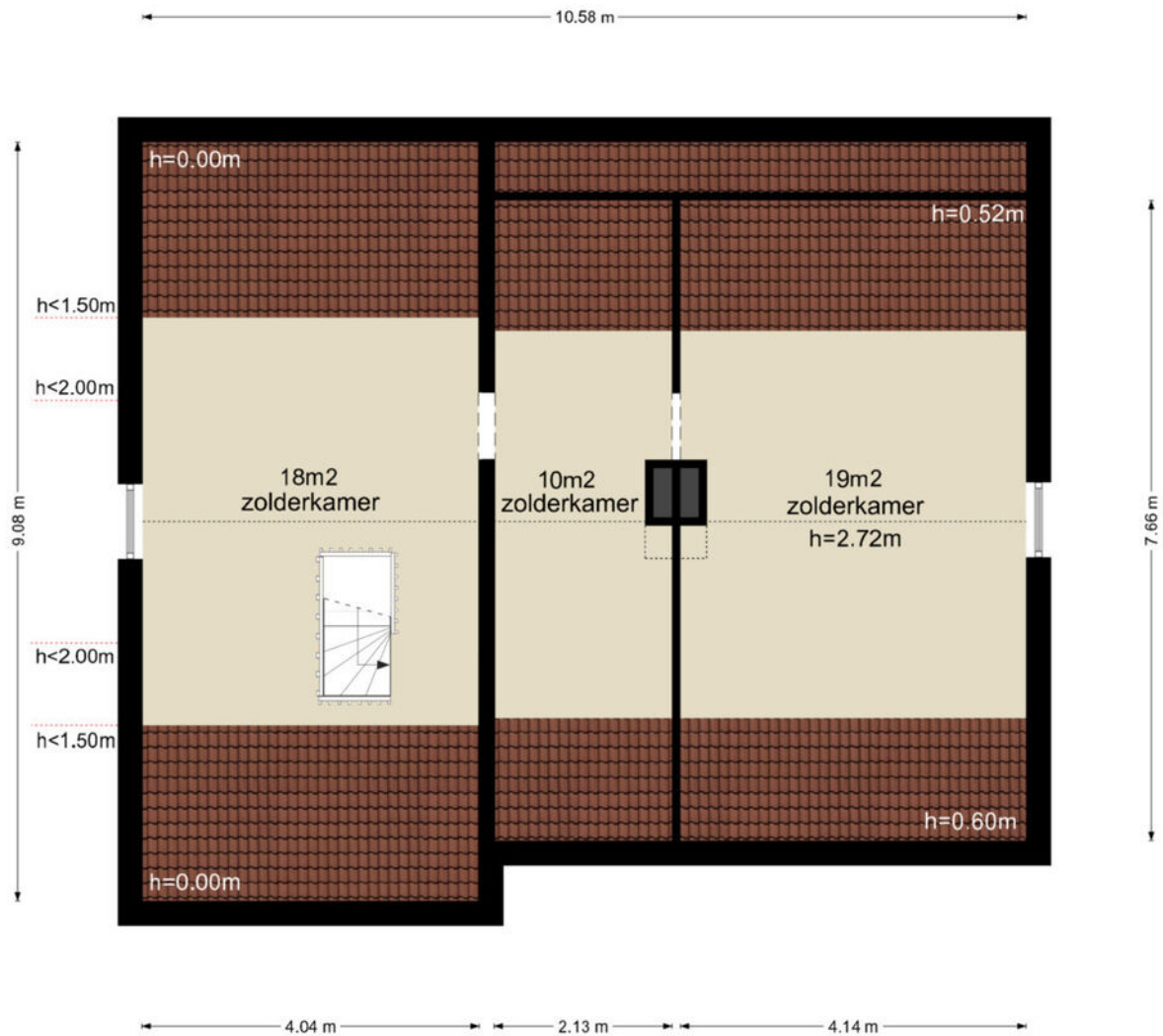
Baarnseweg 66 - Den Dolder Eerste Verdieping
